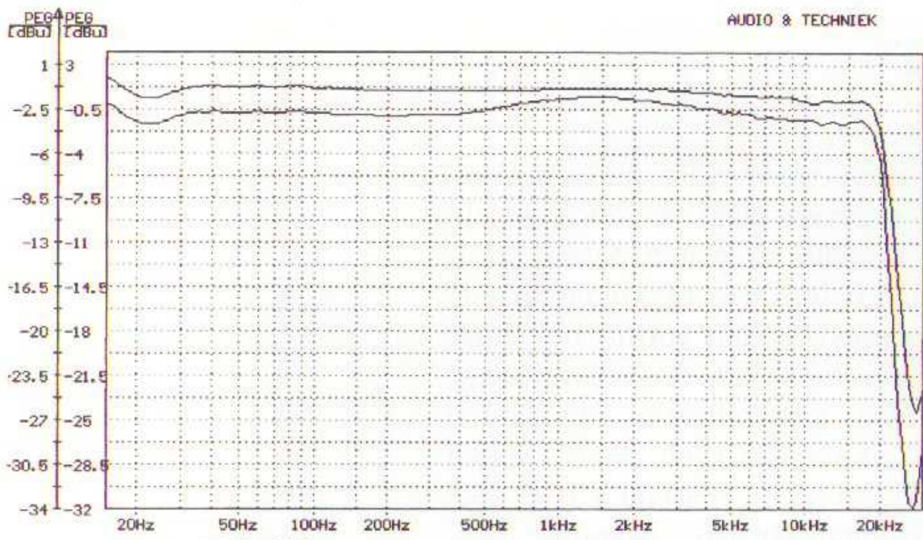
Akai DX-57
